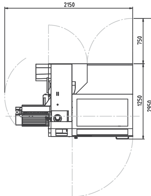
Vista en planta (Dimensiones en mm)
